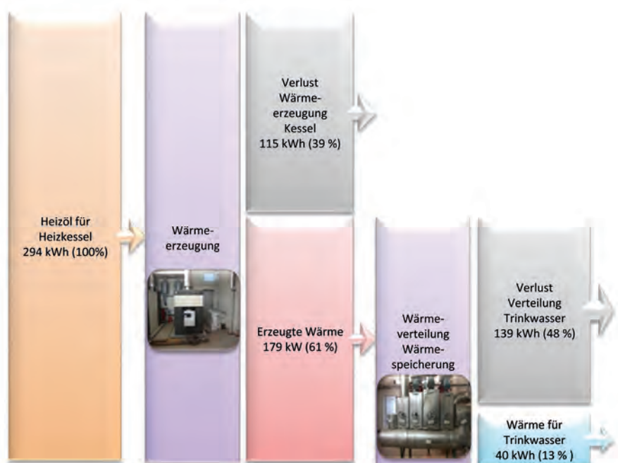
Bild 1: Energieflussbild Trinkwassererwärmung.
