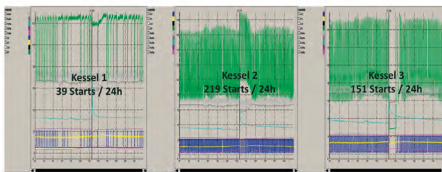
Bild 9: Betriebsverhalten der Heizkessel vor Optimierung.
