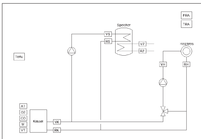
Bild 6: Fühlerschema einer Kesselanlage mit Warmwasserbereitung.
