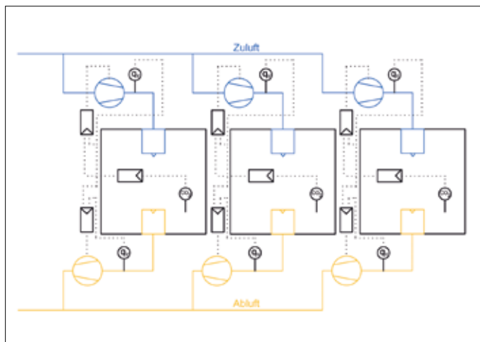
Abbildung 3: dVt-Systemvariante „Einzelraumversorgung (V1a)“
